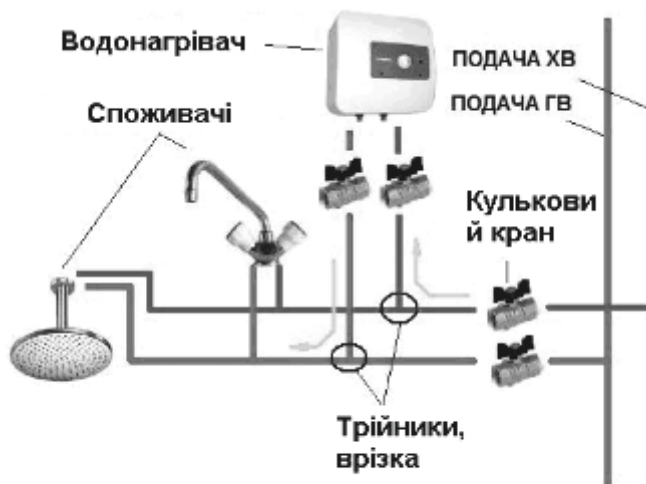
Схема під'єднання проточного водонагрівача
