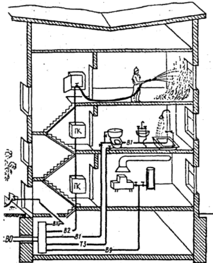
Системи внутрішніх водопроводів:
