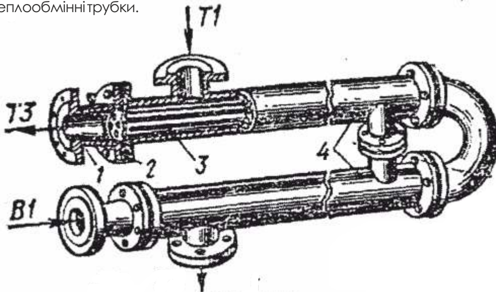
Водяний швидкісний секційний водонагрівач: 1 – вхідний патрубок; 2 – трубні решітки; 3 – труби; 4 – корпус
