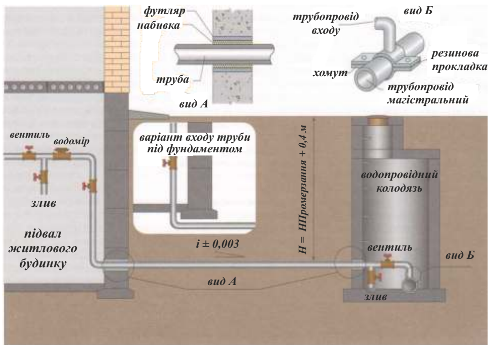
Схема вводу і водомірного вузла в будинку
