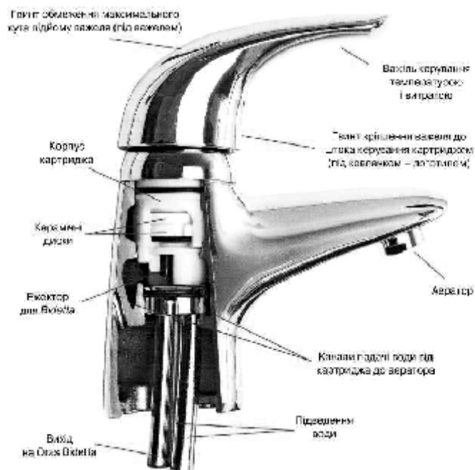
Загальна будова змішувача води (одноважільний)
