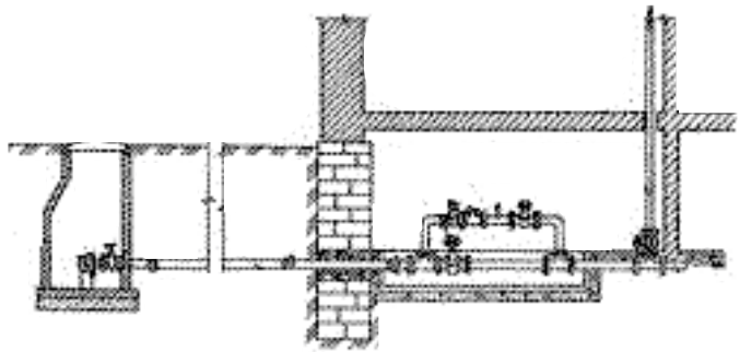
Схема вводу і водомірного вузла в будинку
