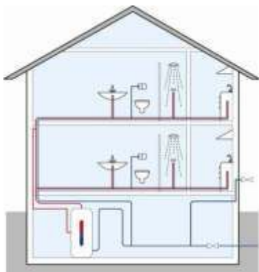
Трійникова тупикова система розведення
