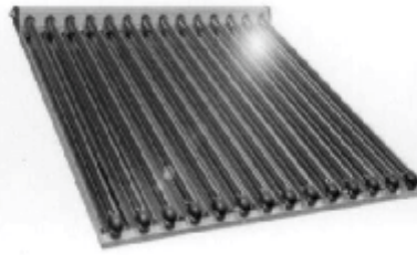
вакуумні лампові колектори з прямим потоком або суха тепла труба
