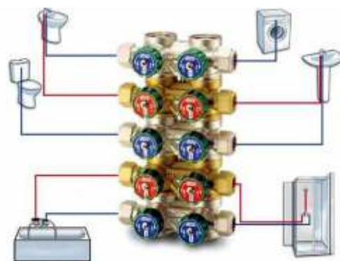
Колектор для холодного та гарячого водопостачання в одній шафі
