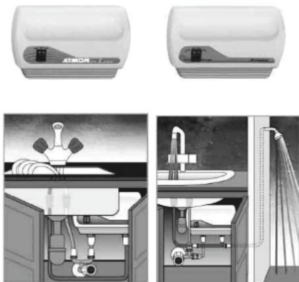
Розміщення проточного водонагрівача
