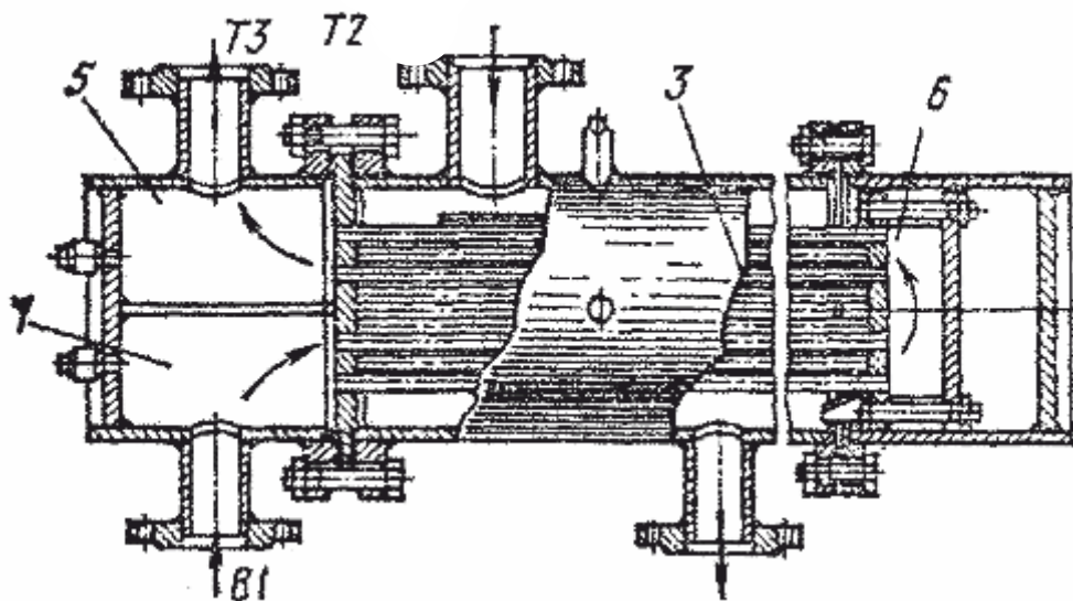
Пароводяний швидкісний водонагрівач 3 – труби; 5-7 – камери
