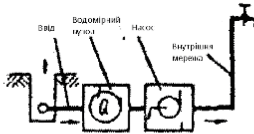
Схема з обладнанням для підвищення тиску
