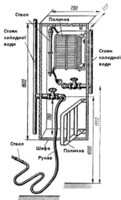
Спарений пожежний кран
