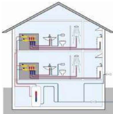
Променева або колекторна система розведення
